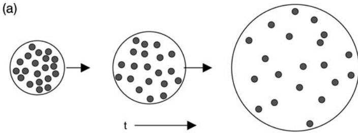
Expandierendes Universum konstanter Masse/Energie
