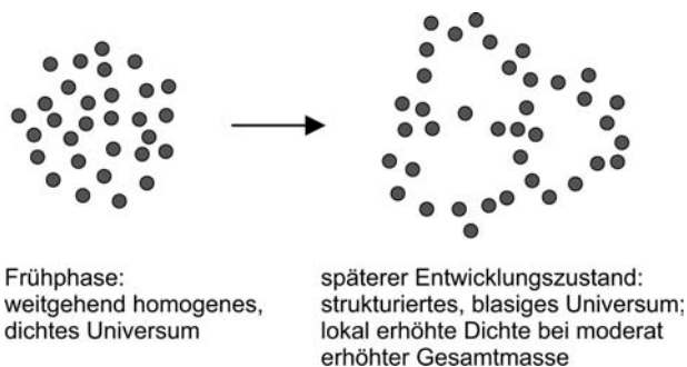
Abb. 34 Annähernde Erhaltung der regionalen Materiedichte in einem inhomogen werdenden Universum bei quadratisch sinkender mittlerer Dichte.
